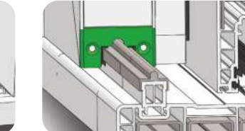
ALT SÜRME KAPAĞI sayesinde sürme kanat kapamanın manuel olarak ray şeklinde kesilmesine gerek kalmadan estetik görünüm sağlanırken kapamanın raya sürme riski ortadan kaldırılmıştır.
